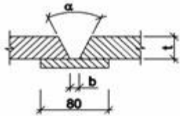
V-ZVAR S PODLOŽKOU t < 4 mm b = 4 až 7 mm \alpha = 20^\circ
