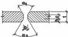
X - ZVAR t = 8 až 10 mm h = t / 2 b = 2 až 3 mm c = 1 až 2 mm \alpha_1 = \alpha_2 = 60^\circ
