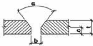
NEPODLOŽENÝ V-ZVAR t = 3 až 20 mm b = 2 až 3 mm c = t až 2 mm \alpha = 60^\circ
