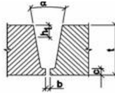
PODLOŽENÝ U-ZVAR t > 40 mm b = 0 až 1 mm c = 3 až 4 mm l_q = t / 4 \alpha = 20^\circ
