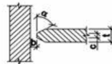
K-ZVAR t = 12 až 40 mm b = 1 až 3 mm c = 1 až 2 mm \alpha = 50^\circ
