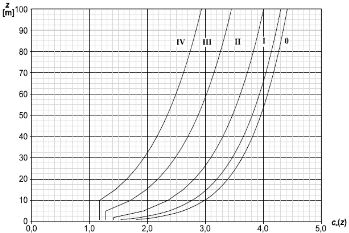
Grafy súčiniteľa vystavenia vetru c_e(z) pre c_0 = 1,0 , k_r = 1,0
